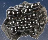
Hematiet/Hematite
