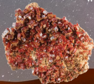
Vanadiniet/Vanadinite
